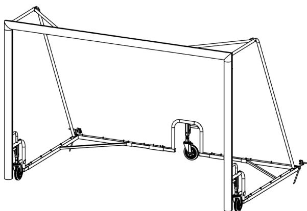
MONTERINGSANVISNING UNISPORT LYFT 3x2m / 3x1,5m Fotbollsmål
